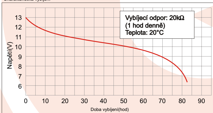
Charakteristika vybíjení
